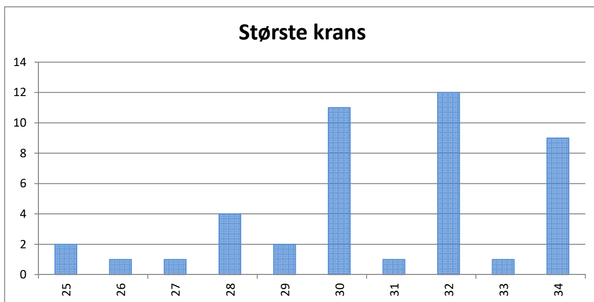
Figur 18 Største krans bagpå
